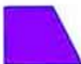
TRAPEZIUM
